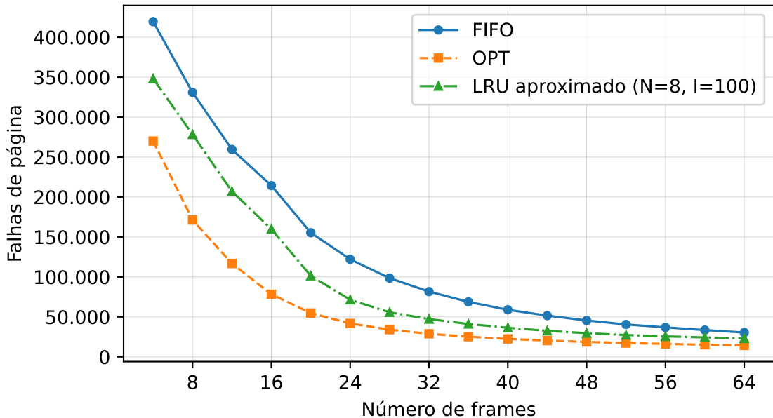
swim: falhas de página por política
