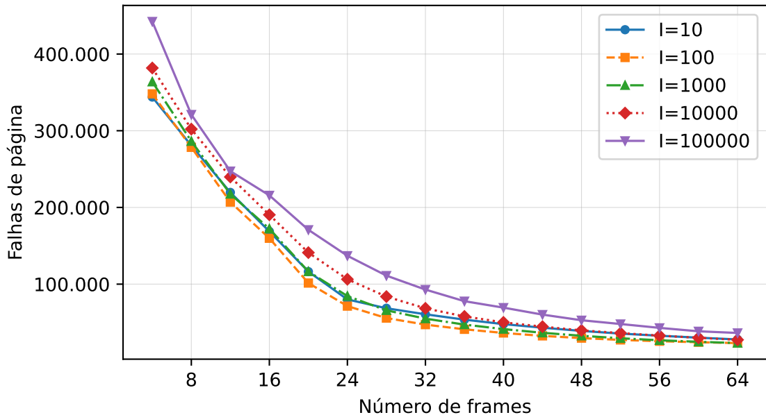
swim: LRU aproximado variando l (N=8)
