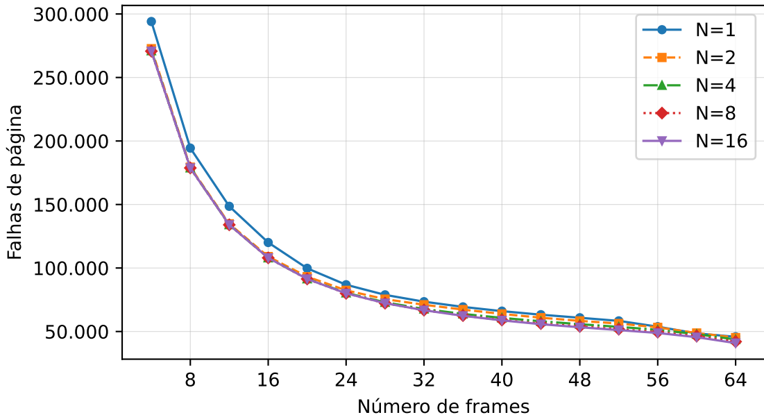
sixpack: LRU aproximado variando N (I=100)
