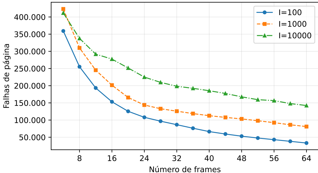
swim: LRU aproximado variando I (N=8)
