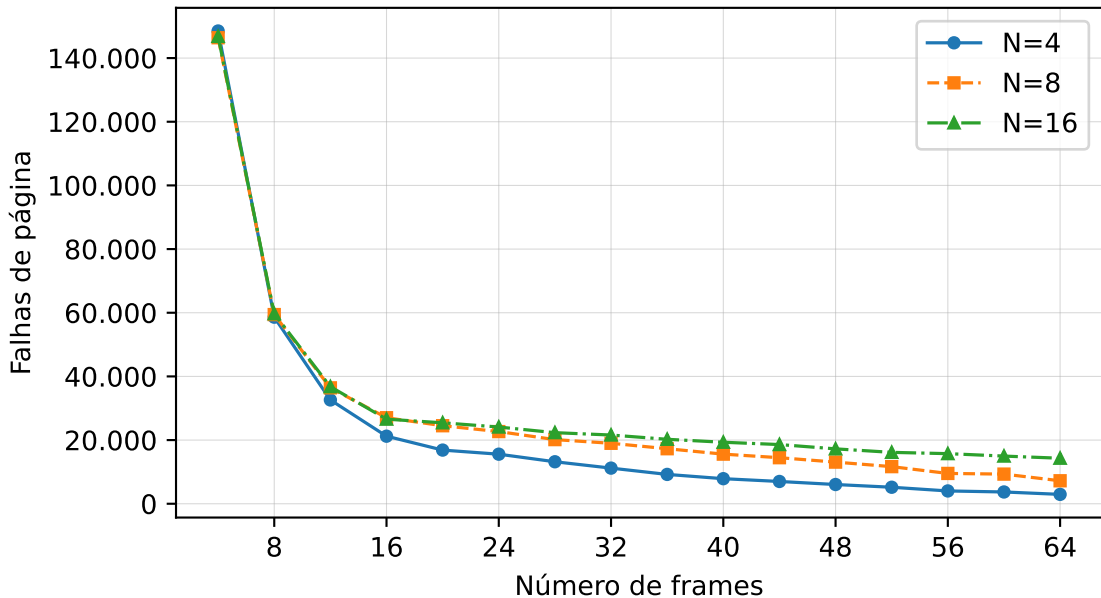
bzip: LRU aproximado variando N (l=1000)
