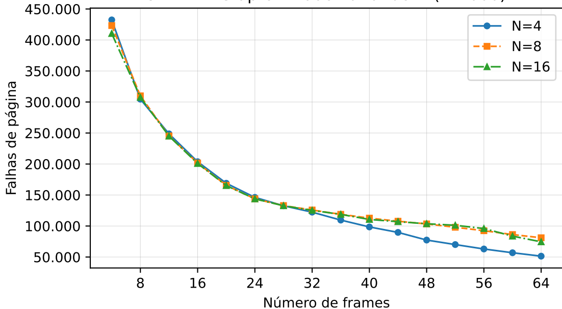
swim: LRU aproximado variando N (I=1000)
