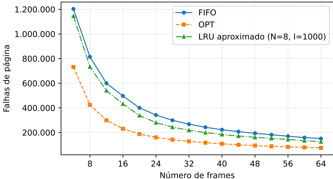
bigone: falhas de página por política
