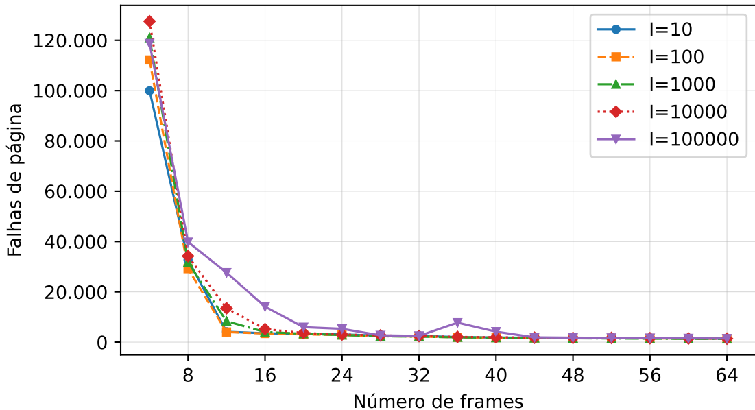
bzip: LRU aproximado variando l ( N=8 )
