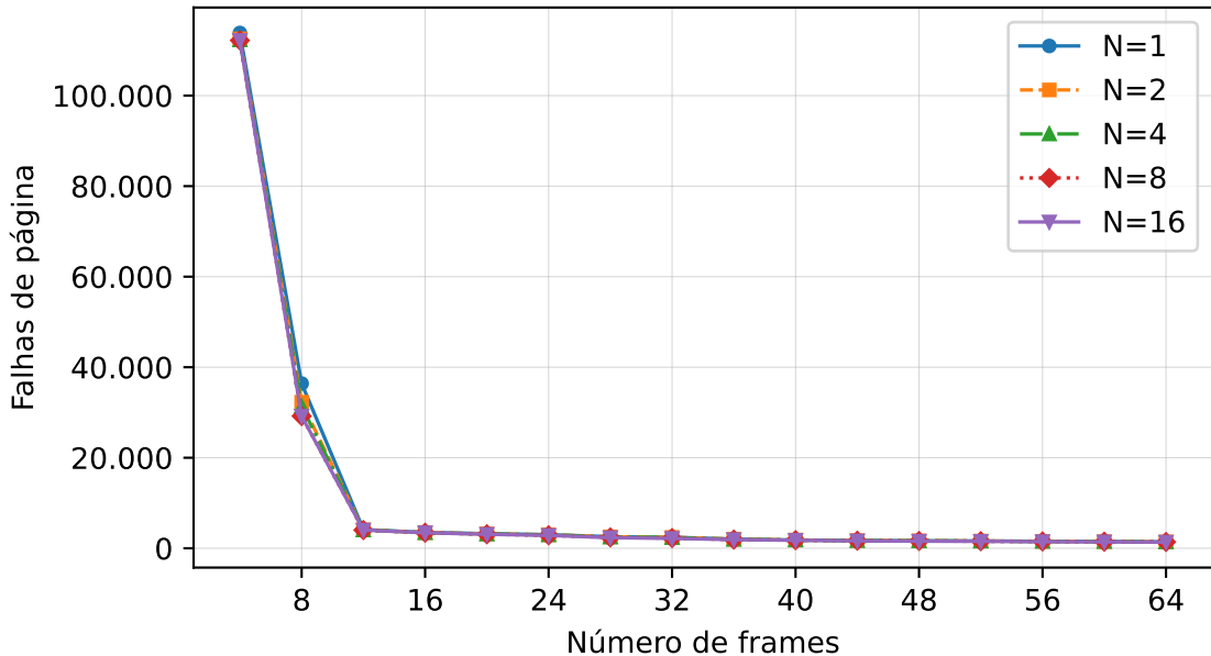
bzip: LRU aproximado variando N (l=100)
