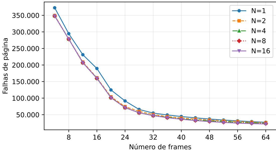
swim: LRU aproximado variando N (I=100)
