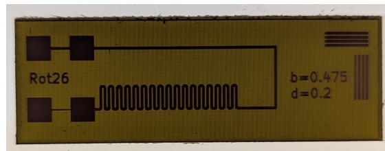
Abbildung 1.10 Fertig produzierte Leiterplatte.
