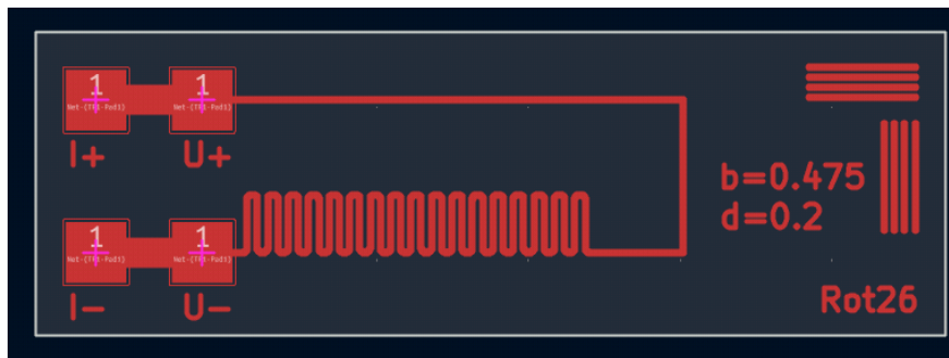
Abbildung 1.1 KICAD Leiterplattendesign eines Leiterbahnwiderstand mit 200 mΩ
