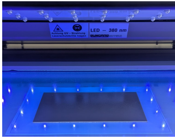
Abbildung 1.3 Erstellung des Photoresist durch schwarzlichtbeleuchtung des Photolacks unter der Schablone.
