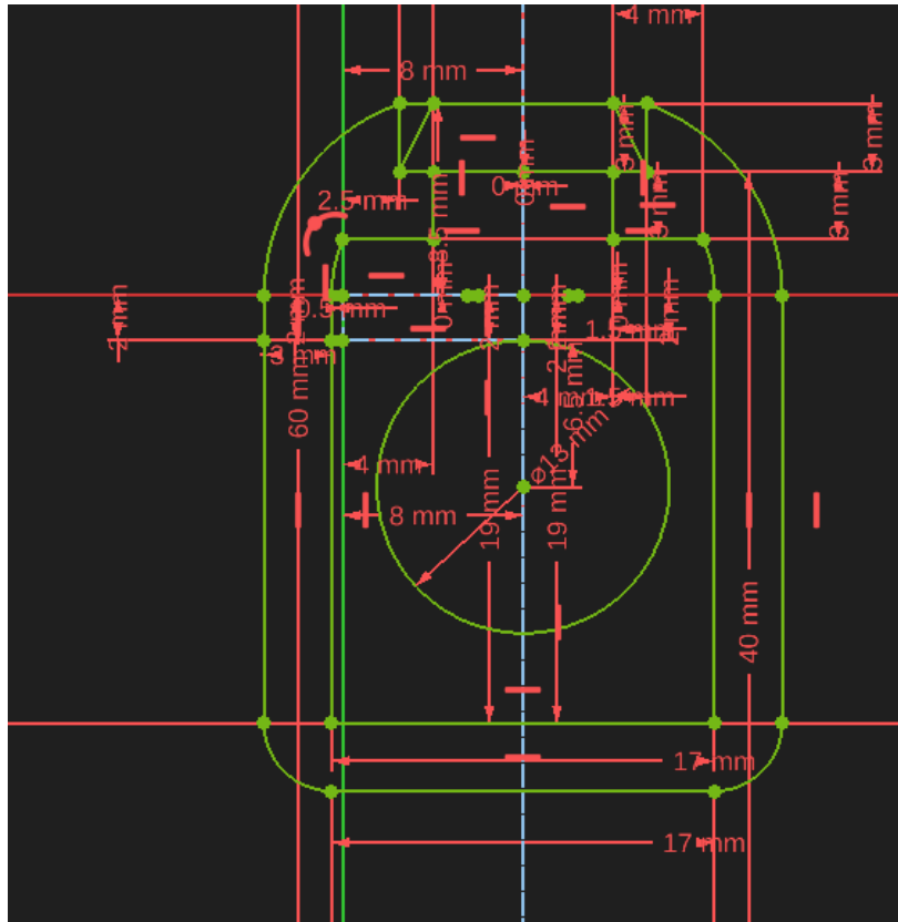
Abbildung 2.5 Skizze der Frontansicht des Gehäuses mit Symmetrielinie gezeichnet.
