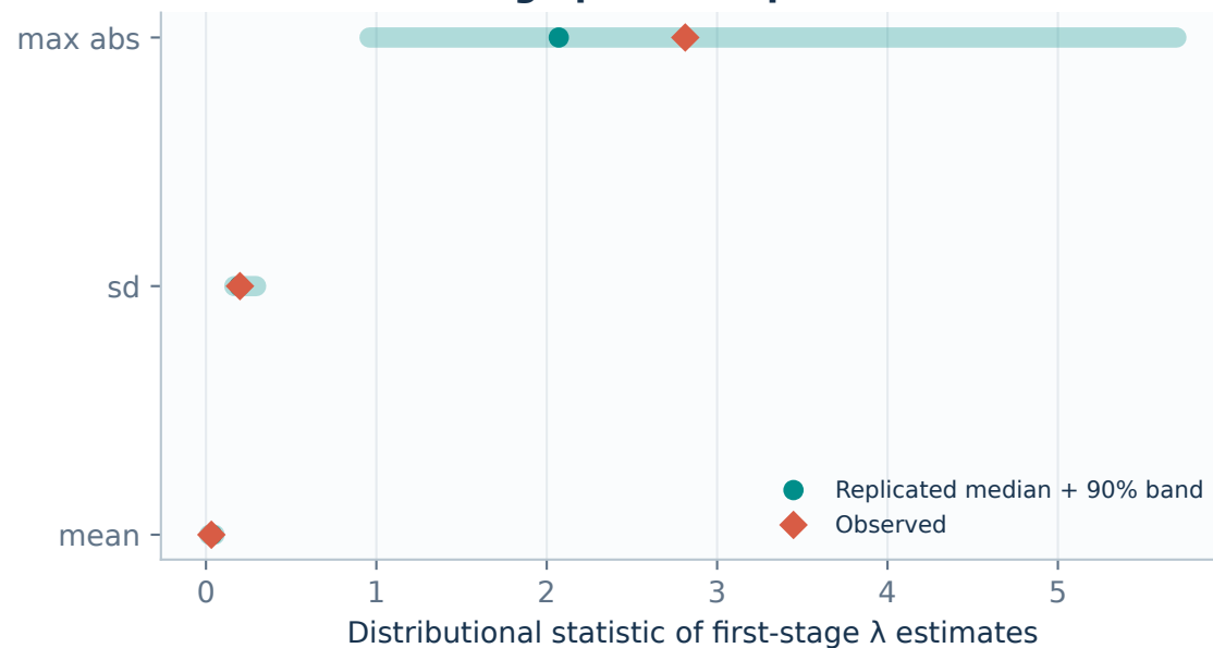
Second-stage posterior predictive check
