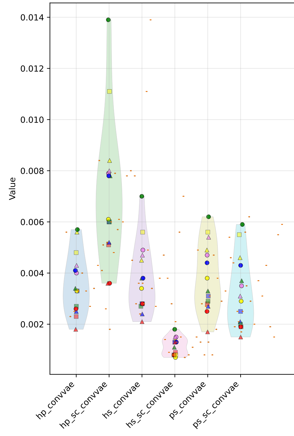
TPR at FPR 1e-4
