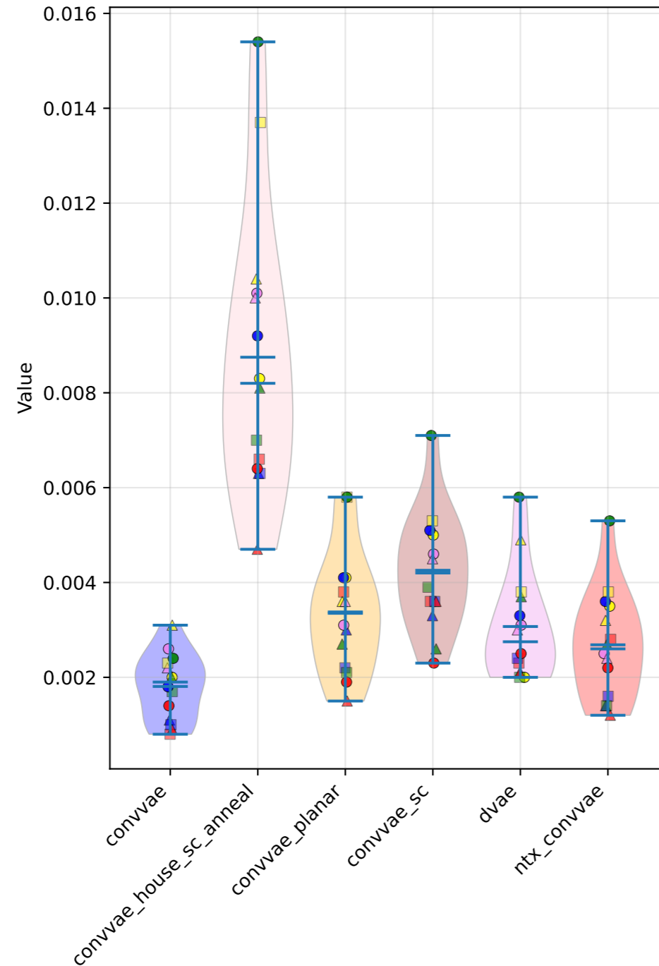
TPR at FPR 1e-4
