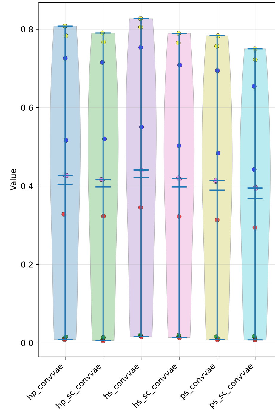
TPR at FPR 1e-2
