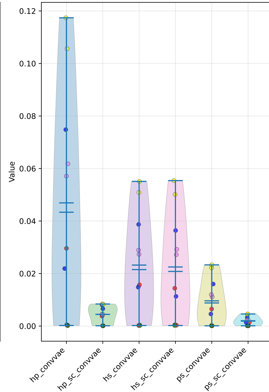
TPR at FPR 1e-4
