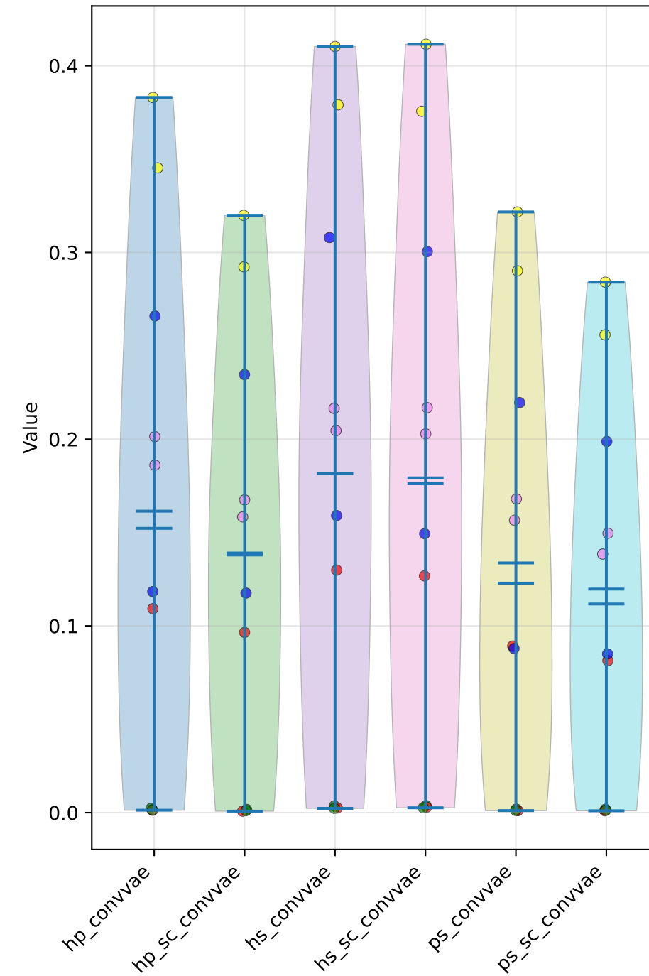
TPR at FPR 1e-3
