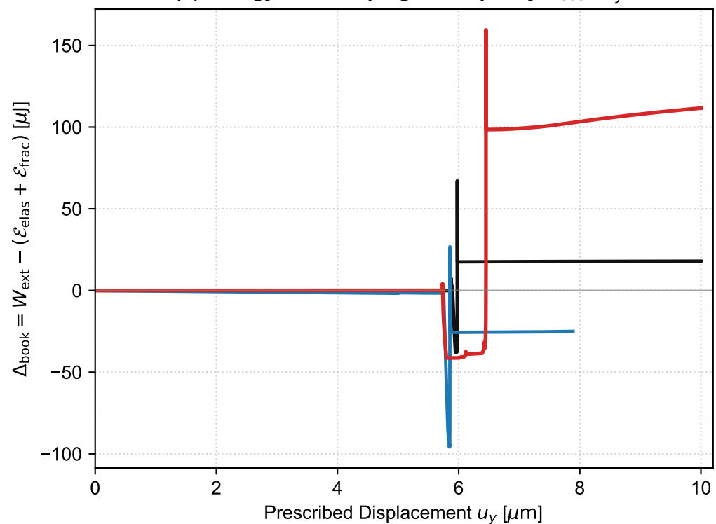
(d) Energy Bookkeeping Discrepancy \Delta_{\text{book}}(u_y)
