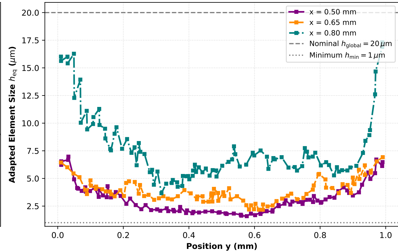
(d) Vertical Profiles: Adapted Sizing h_{eq}(y)
