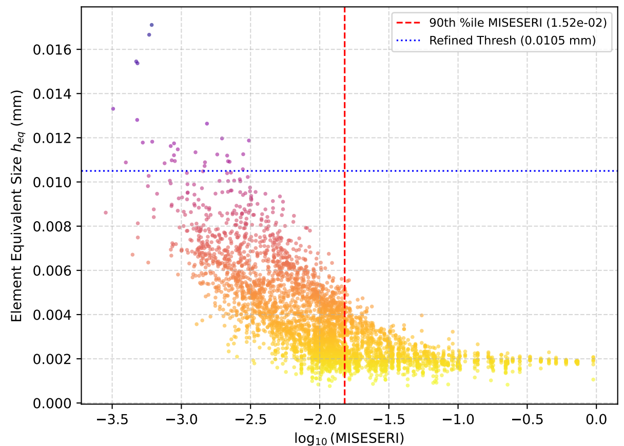
(d) Element Sizing vs Indicator Field (Pearson r = -0.6998 )
