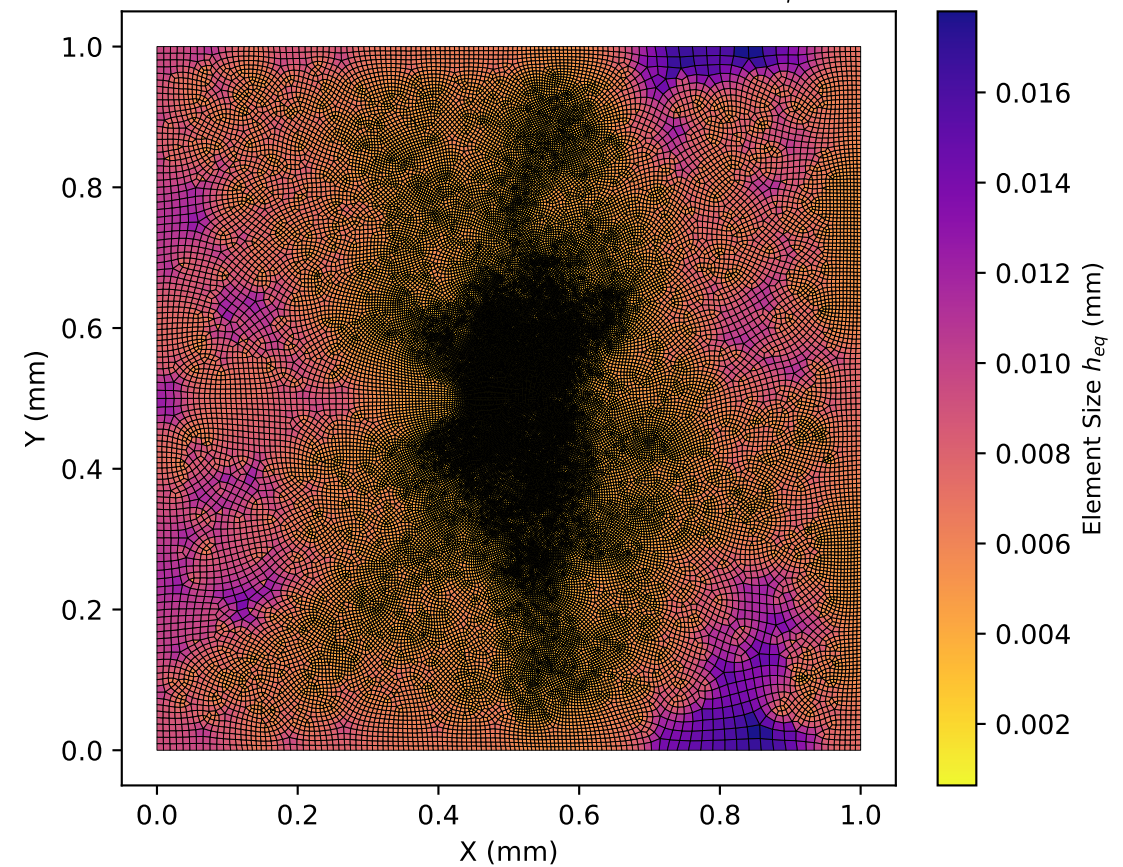
(d) Element Sizing vs Indicator Field (Pearson r = -0.6998 )
