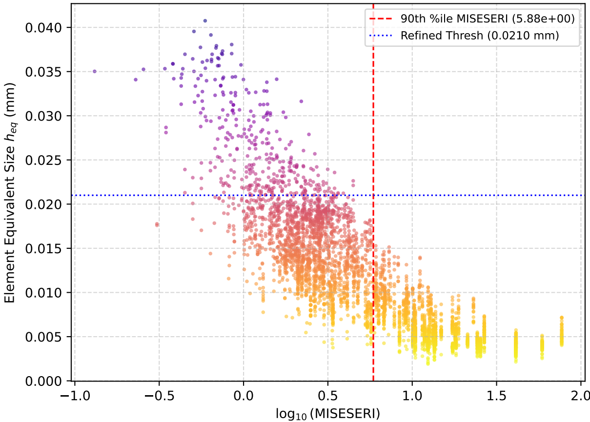
(d) Element Sizing vs Indicator Field (Pearson r = -0.8332 )
