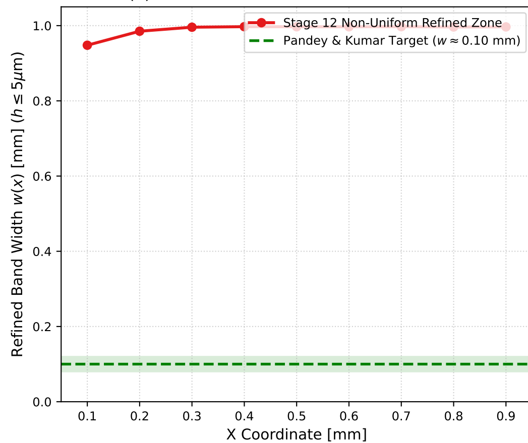
(d) Refined Corridor Width Across Domain
