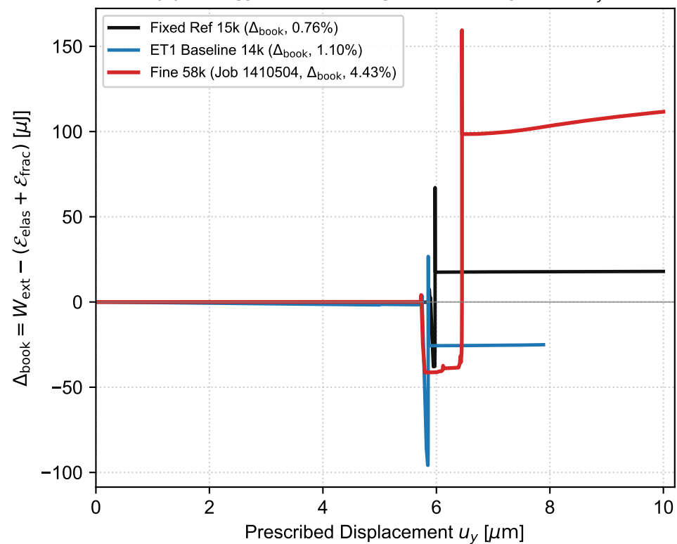
(d) Energy Bookkeeping Discrepancy \Delta_{\text{book}}(u_y)
