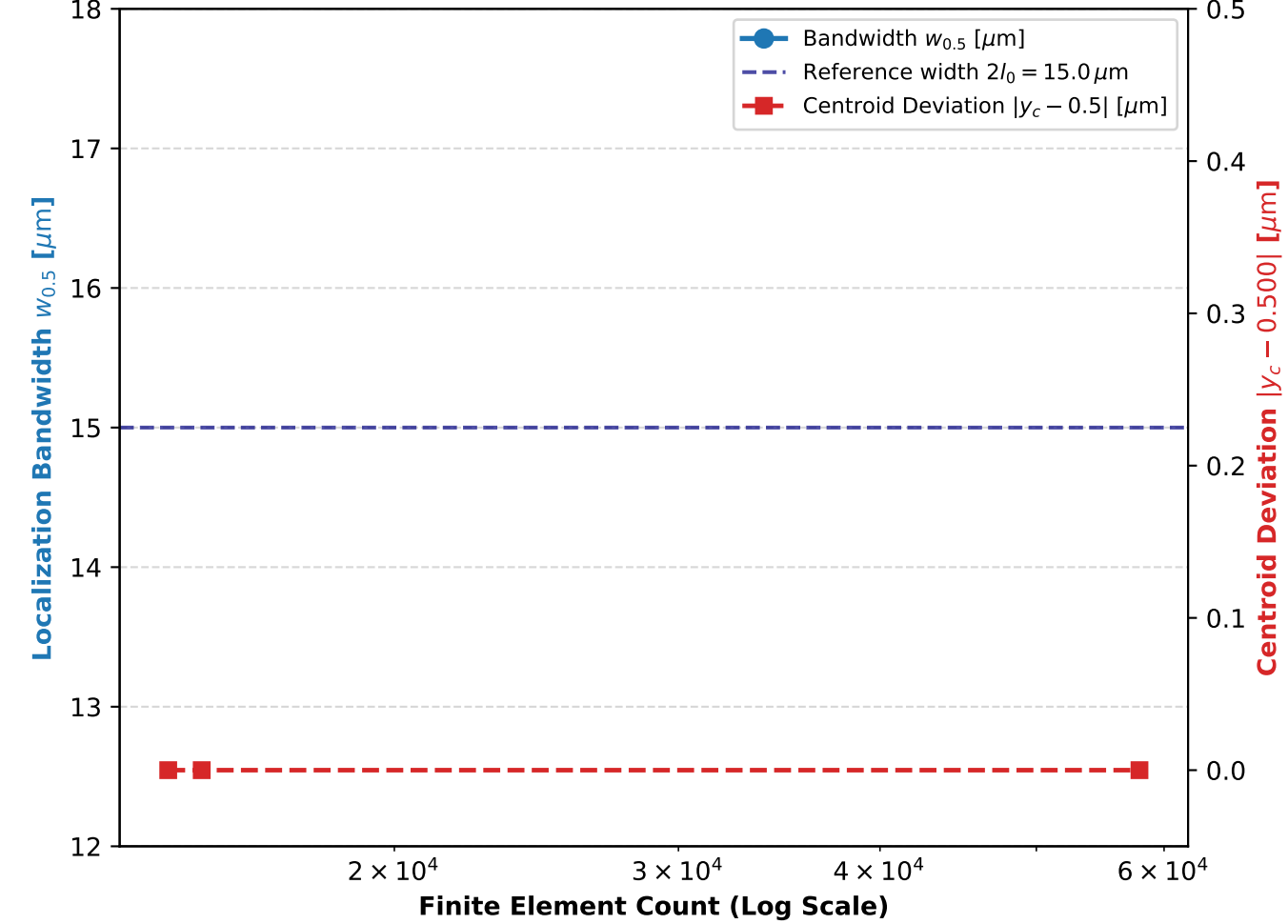
(d) Localization Bandwidth w_{0.5} vs Finite Element Count
