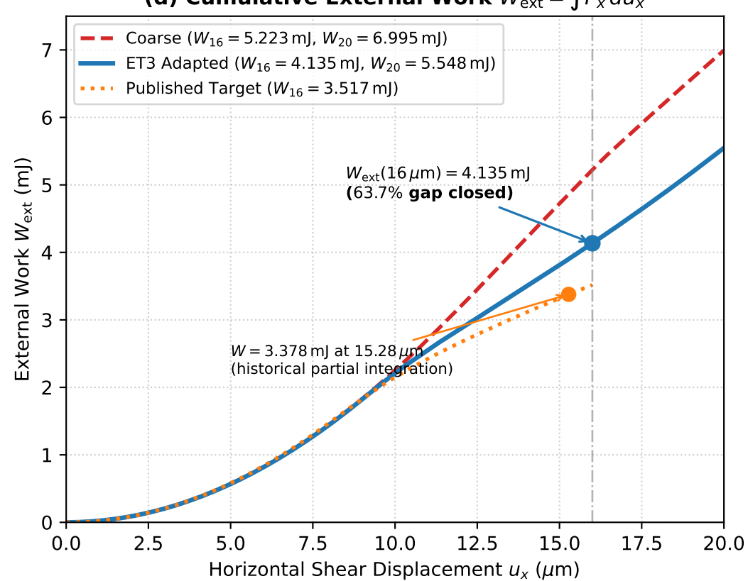
(d) Cumulative External Work W_{\text{ext}} = \int F_x du_x
