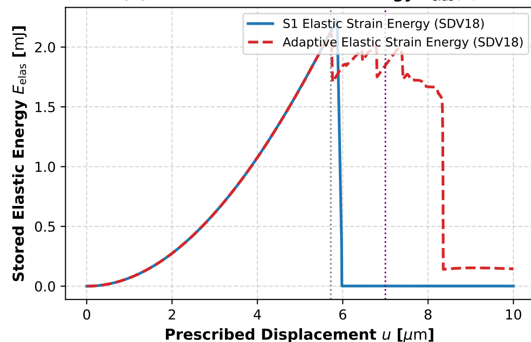
(d) Stored Elastic Strain Energy E_{\text{elas}}(u)
