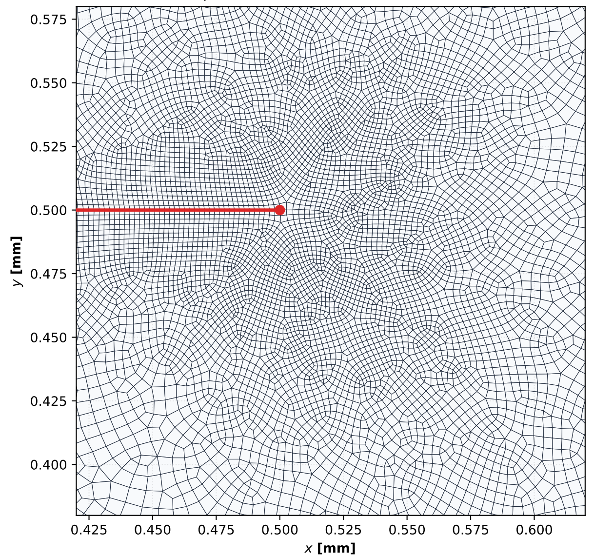
(d) Step-2 Crack-Tip Singularity Zoom
