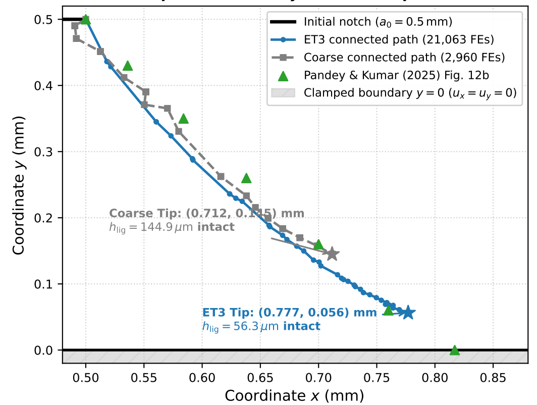
(d) Spatial Crack Trajectories & Tip Arrest
