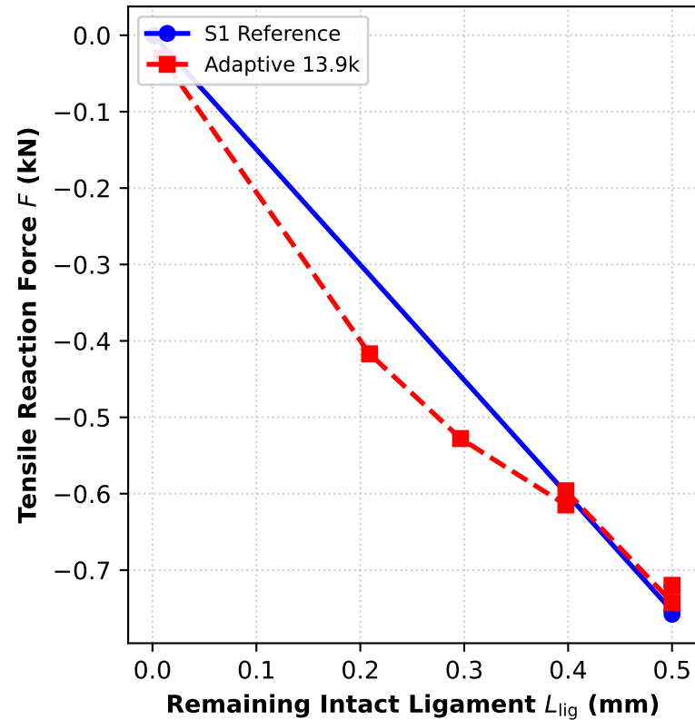
(d) Force vs Remaining Ligament F(L_{\text{lig}})
