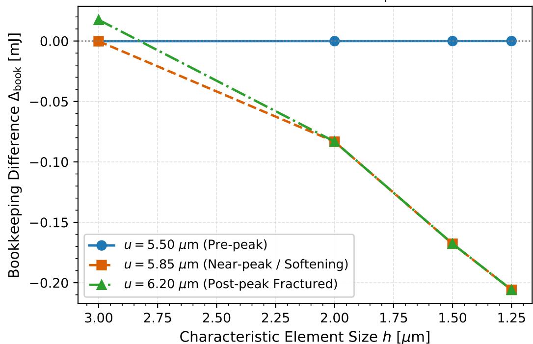
(d) Two-Term Difference \Delta_{\text{book}} \equiv W_{\text{trap}} - (E_{\text{elas}} + E_{\text{frac}})
