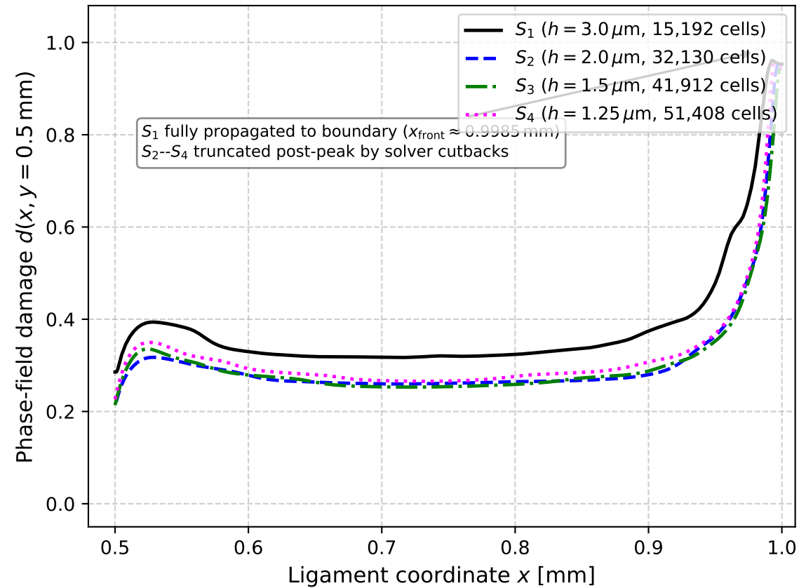
(d) Post-Peak Crack Propagation: u = 6.20 \mu\text{m}
