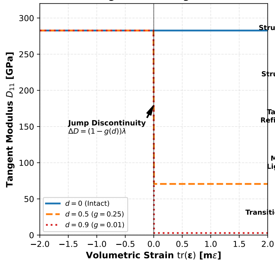
(d) 2D Miehe Algorithmic Tangent Discontinuity
