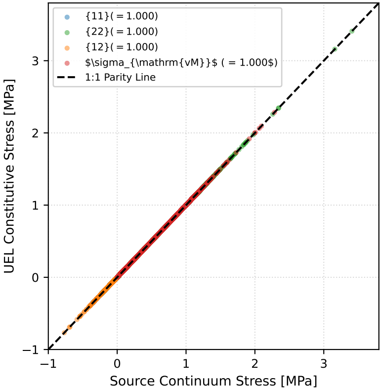
(d) Constitutive Stress Component Parity
