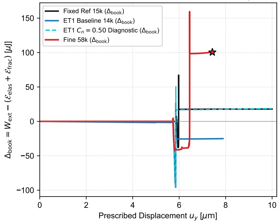
(d) Energy Bookkeeping Discrepancy \Delta_{\text{book}}(u_y)
