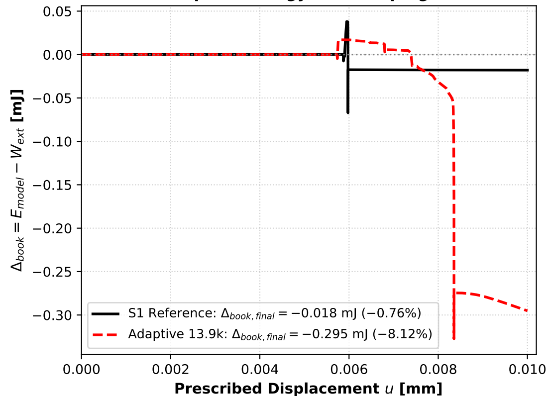
(d) Descriptive Energy Bookkeeping Residual
