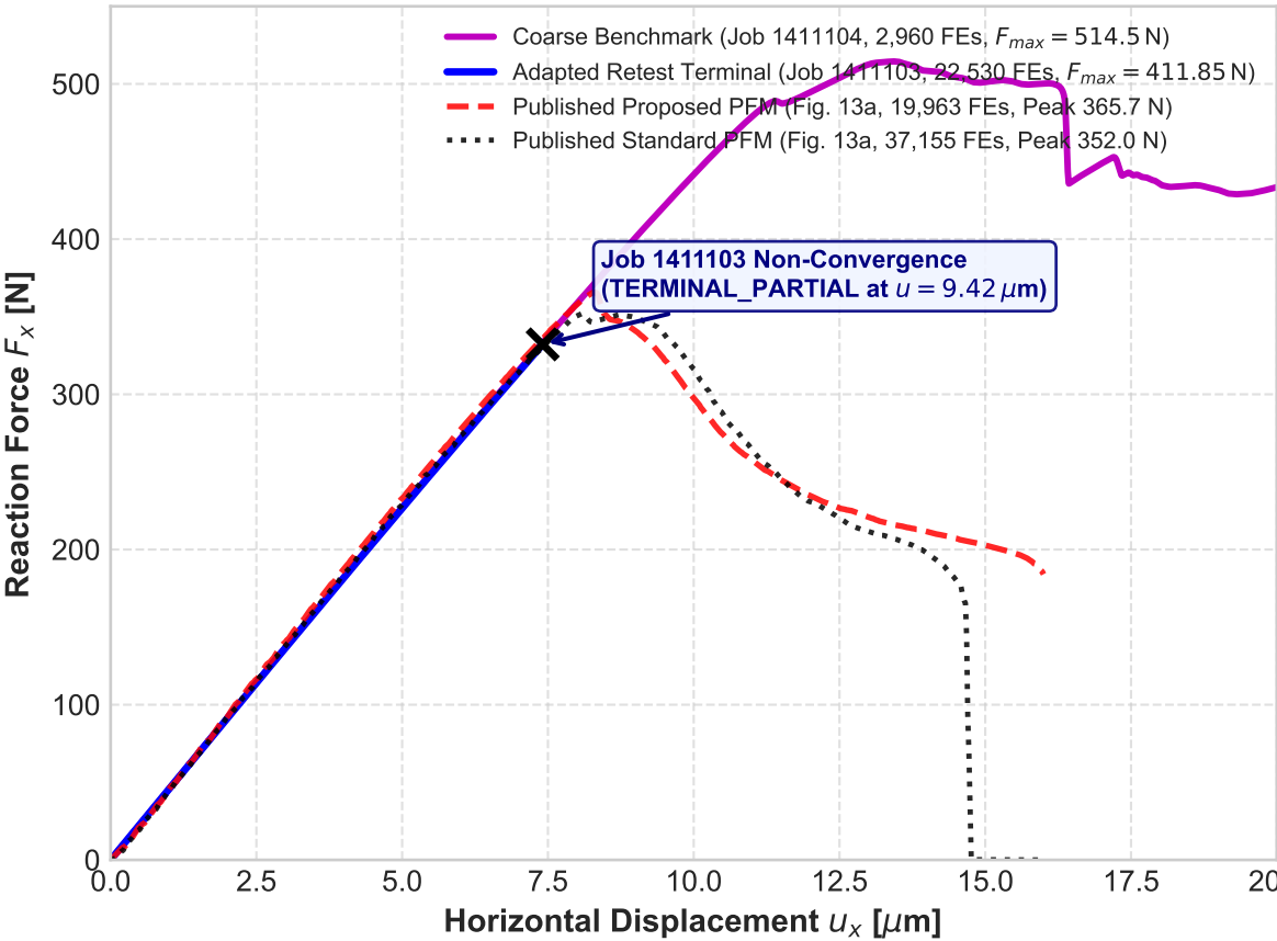
(d) Force-Displacement Response & Solver Execution Benchmark
