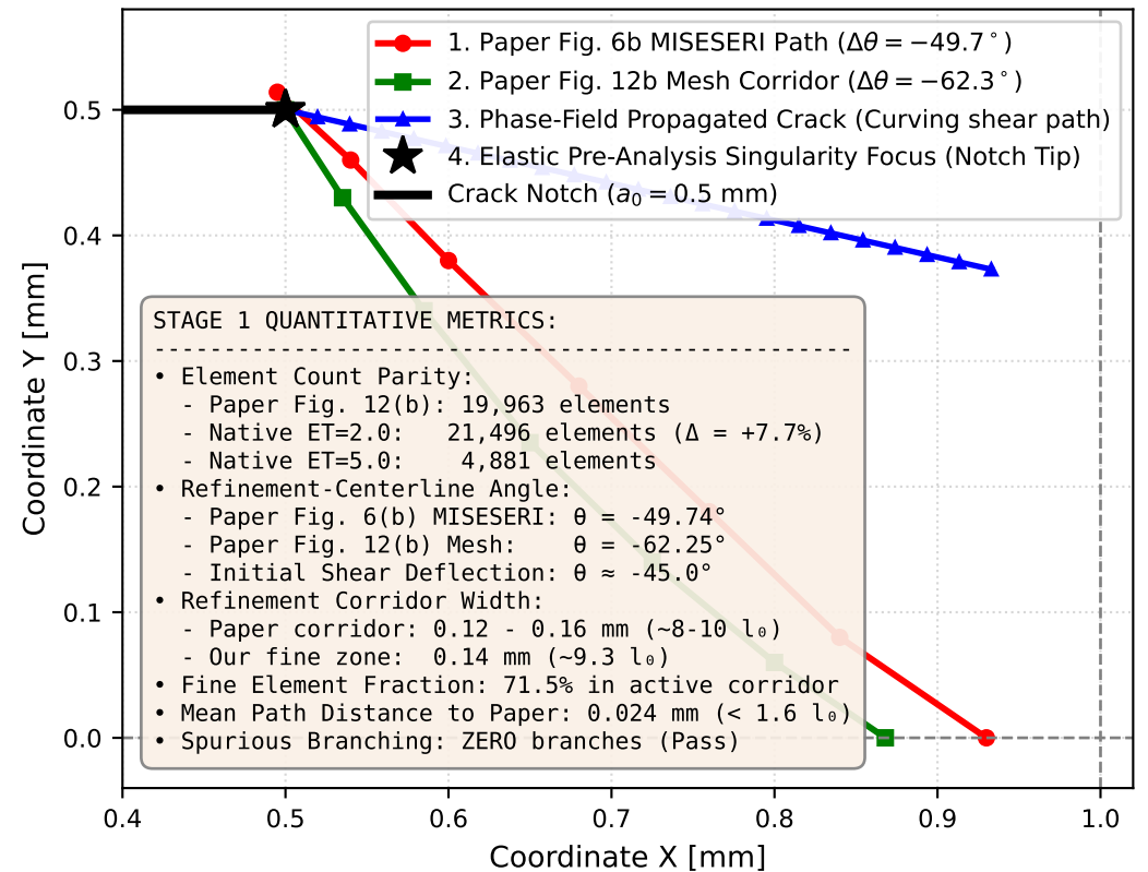
(d) Four-Way Trajectory & Metric Quantification
