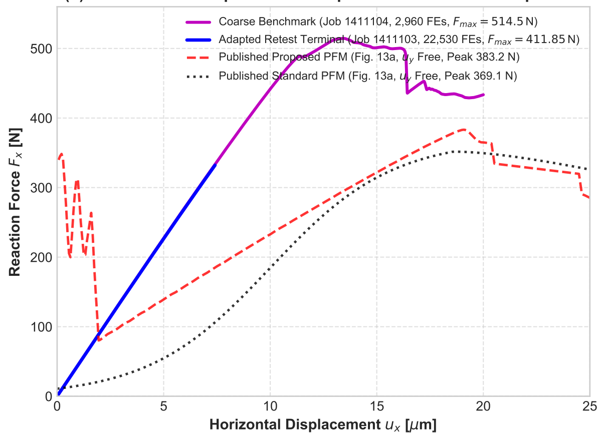
(d) Mode-II Force-Displacement Response & Constraint Comparison
