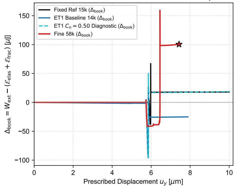
(d) Energy Bookkeeping Discrepancy \Delta_{\text{book}}(u_y)
