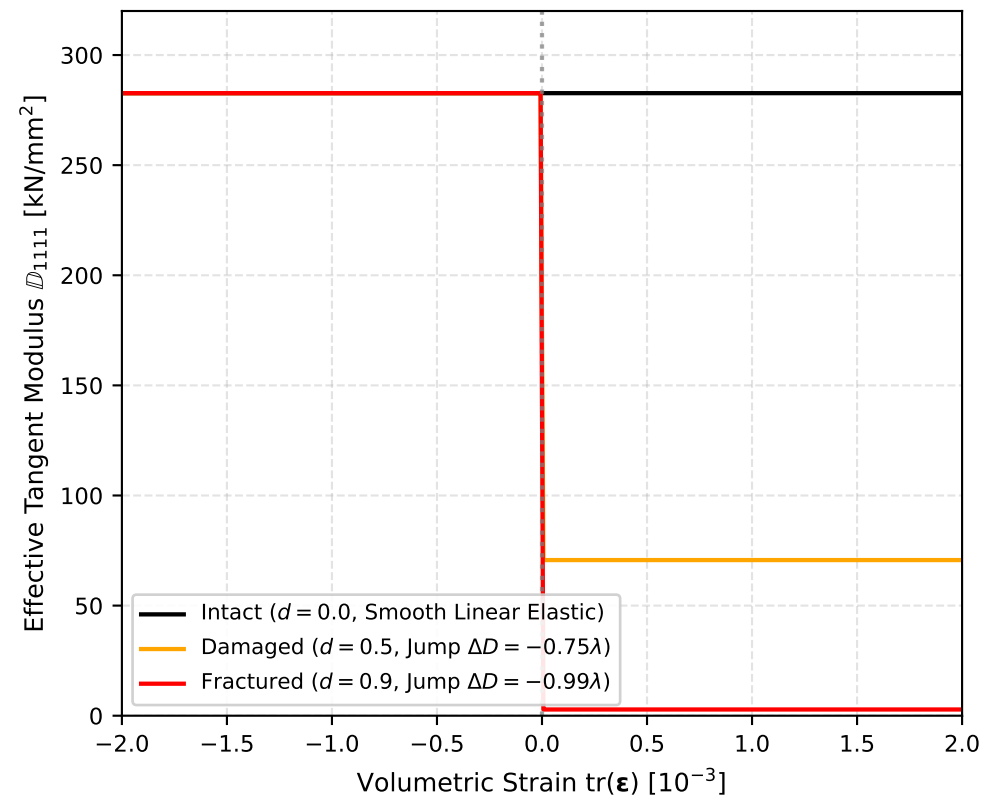
(d) Miehe Spectral Split: Subgradient Jump at \text{tr}(\boldsymbol{\epsilon}) = 0
