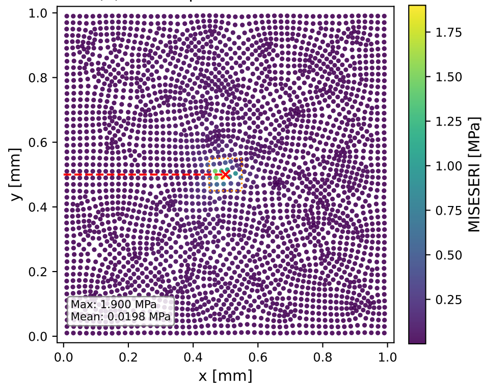
(d) End Step 2: u = 0.0100 mm
