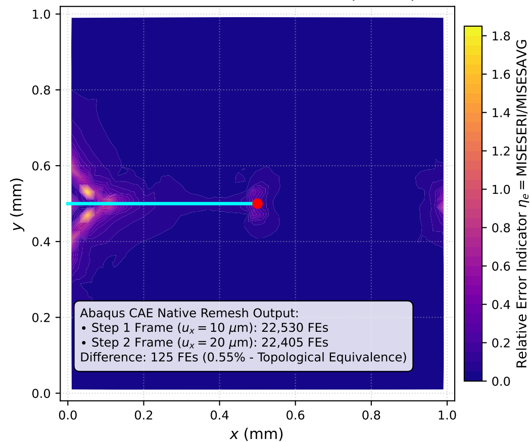
(d) Relative Error Distribution & Sizing Fan Drives Refinement from h = 20 \mu\text{m} \rightarrow 1 \mu\text{m}
