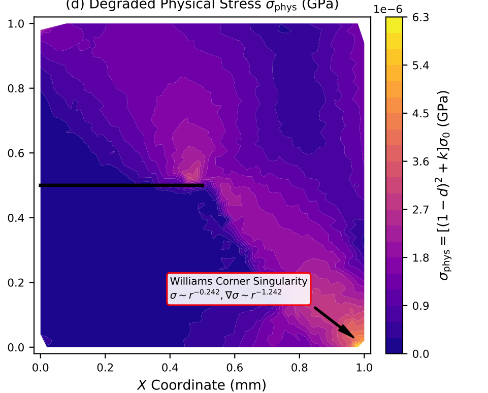
(d) Degraded Physical Stress \sigma_{\text{phys}} (GPa)
