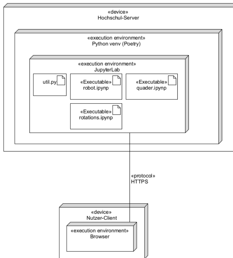
Abbildung 1: Verteilungsdiagramm des Frameworks
