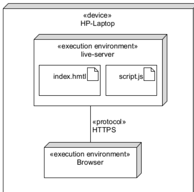
Abbildung 7: Verteilungsdiagramm des Frameworks
