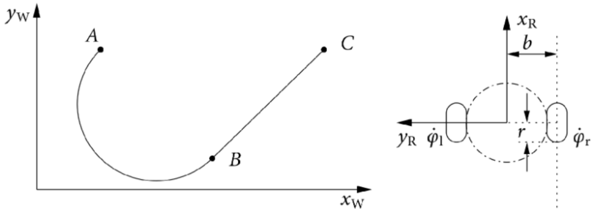
Abbildung 4: Roboter mit Differentialantrieb (Bild aus der Übungsaufgabe)
