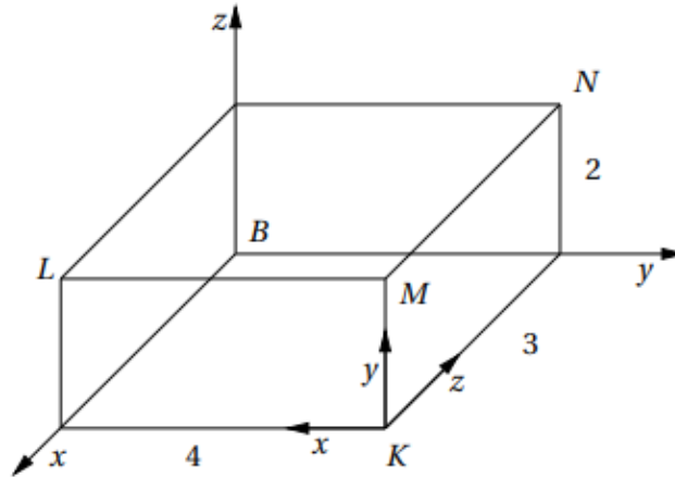
Abbildung 6: Quader aus der Klausuraufgabe
