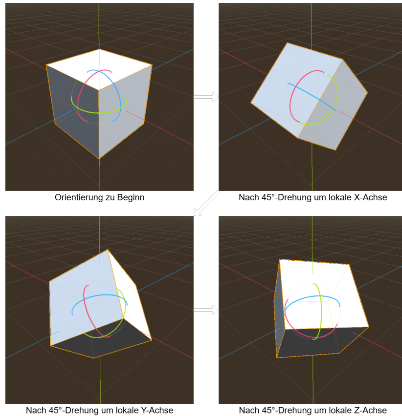
Abbildung 1: Eulerrotation eines Würfels um X, Y und Z in dieser Reihenfolge
