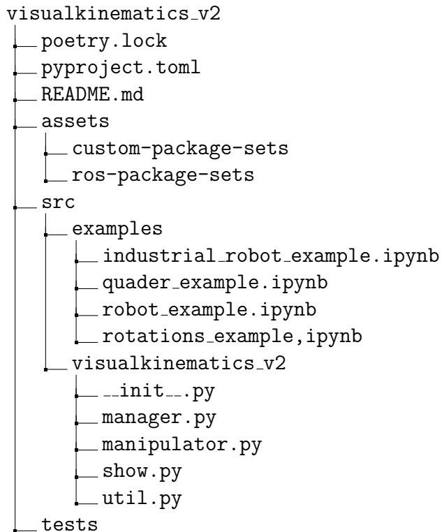
Abbildung 14: Verzeichnisstruktur des Packets visualkinematics_v2
