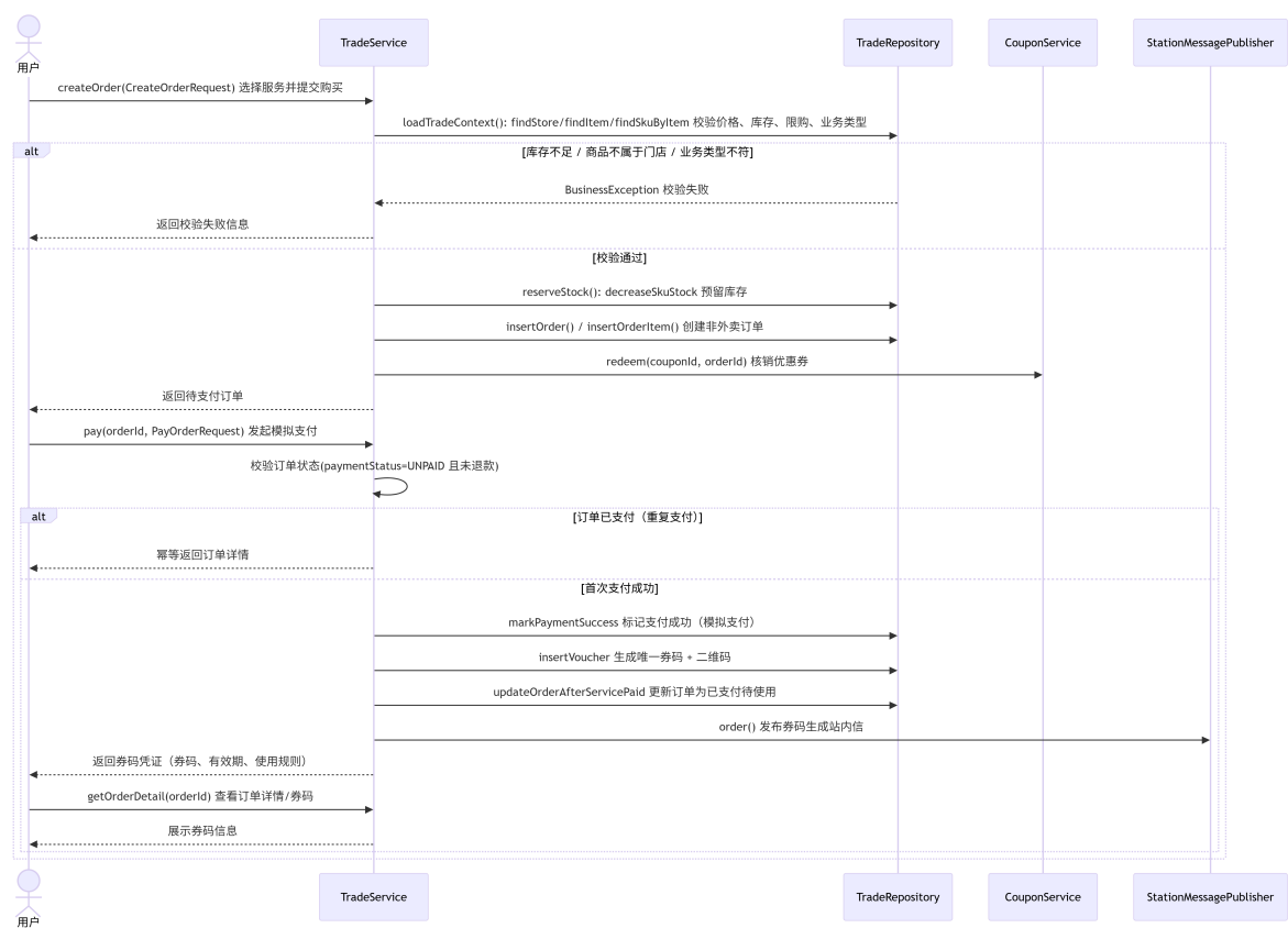
OBJ-SEQ06 非外卖购买出券对象级顺序图。
