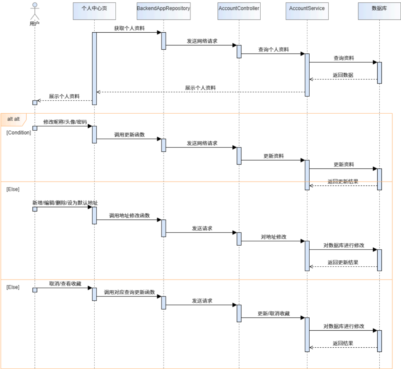
OBJ-SEQ03 用户资料地址收藏对象级顺序图。
