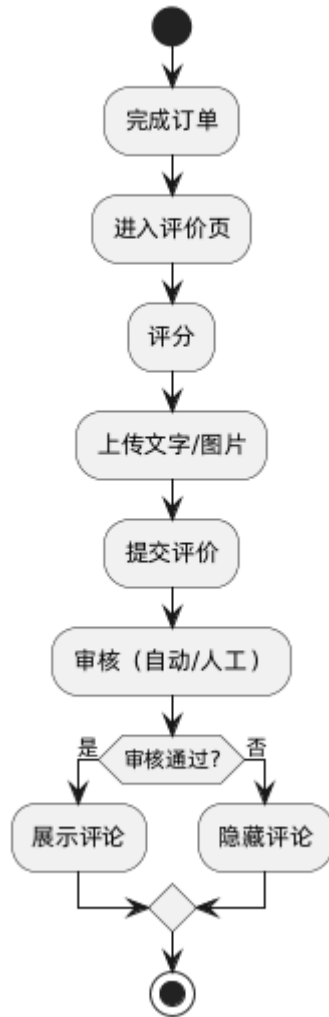
收藏与评价活动图
