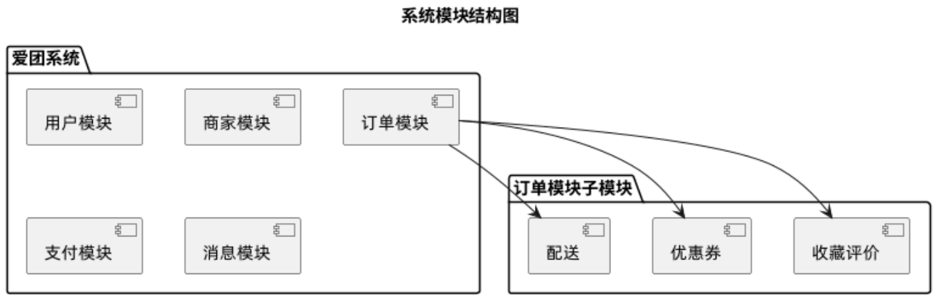
图 2-20 系统模块结构图
