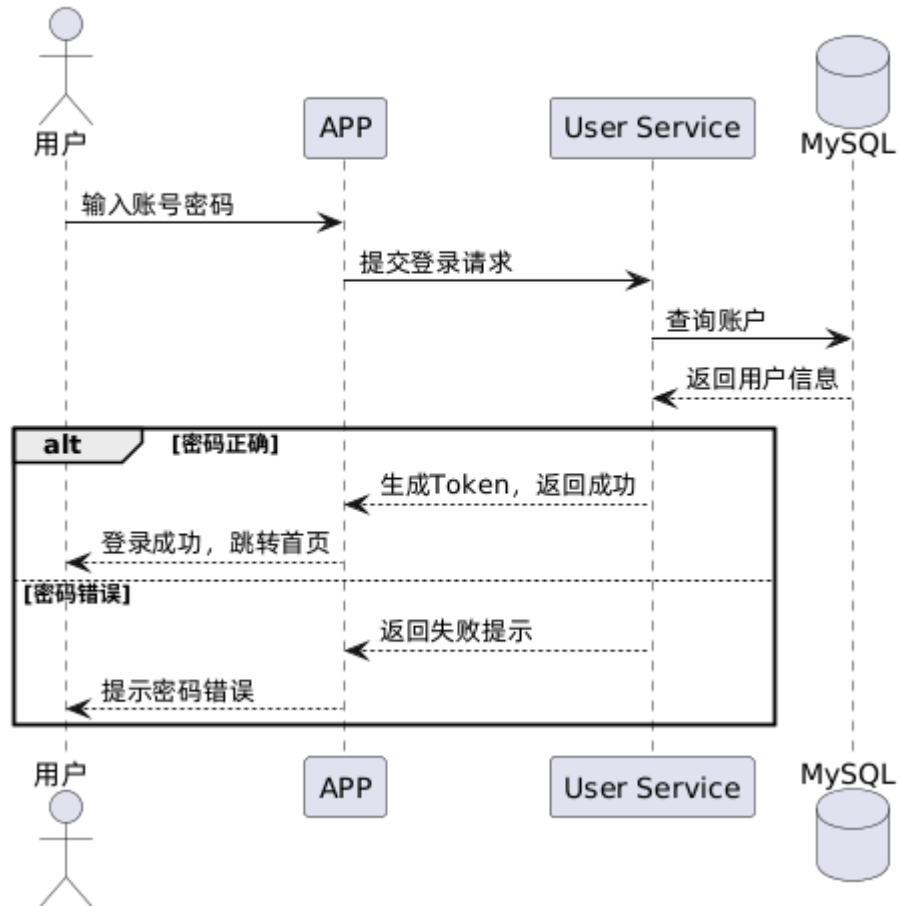
用户登录顺序图
