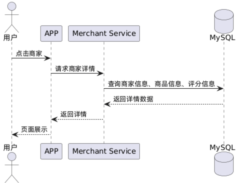
商家详情顺序图
