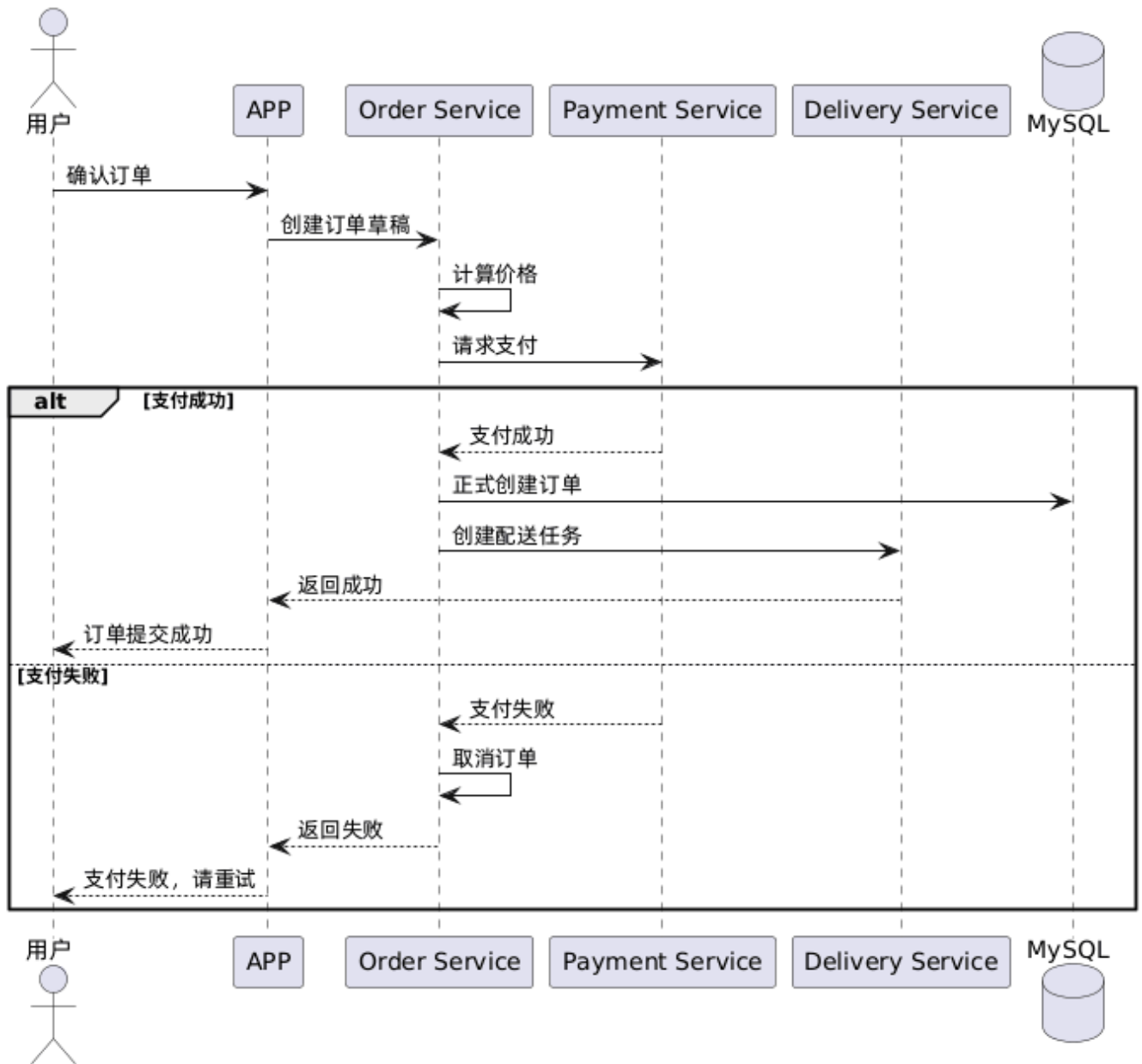
提交订单顺序图（核心流程）
