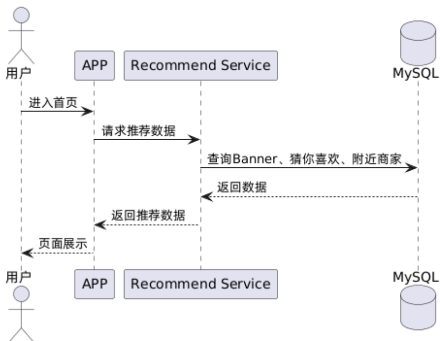
首页推荐顺序图
