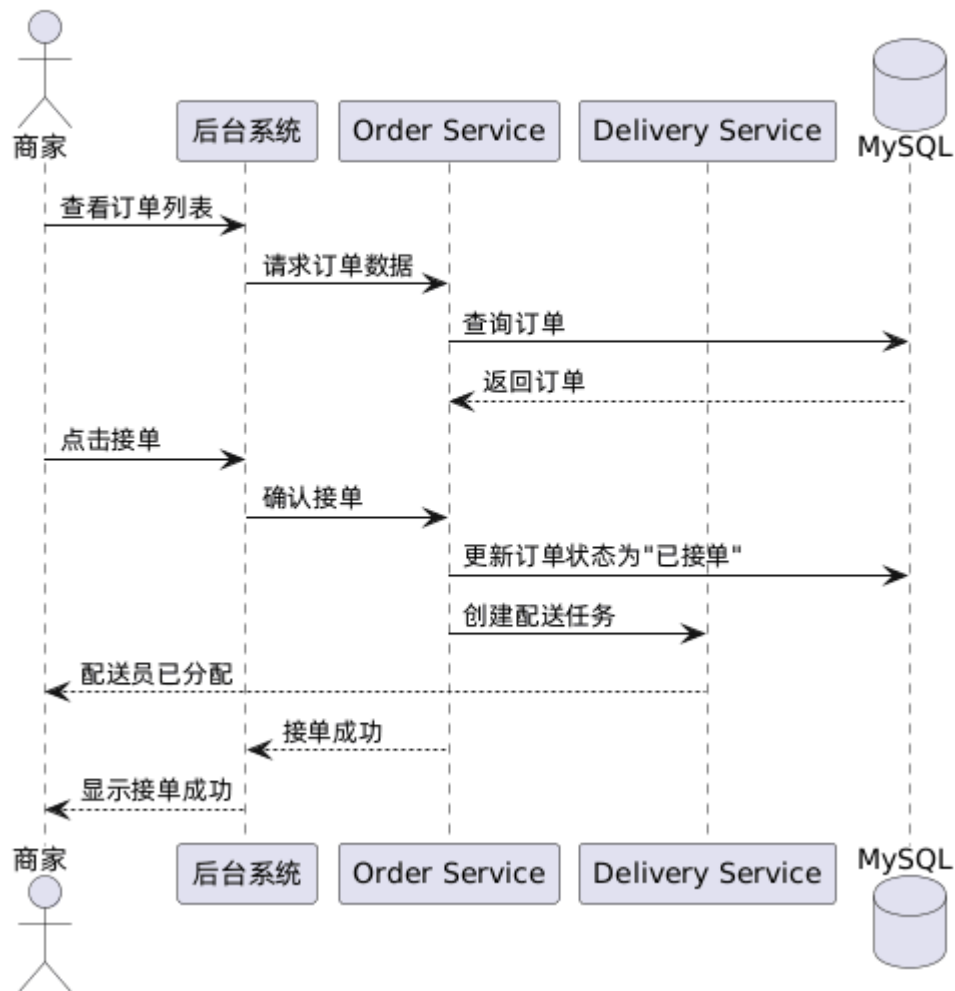
商家处理订单顺序图
