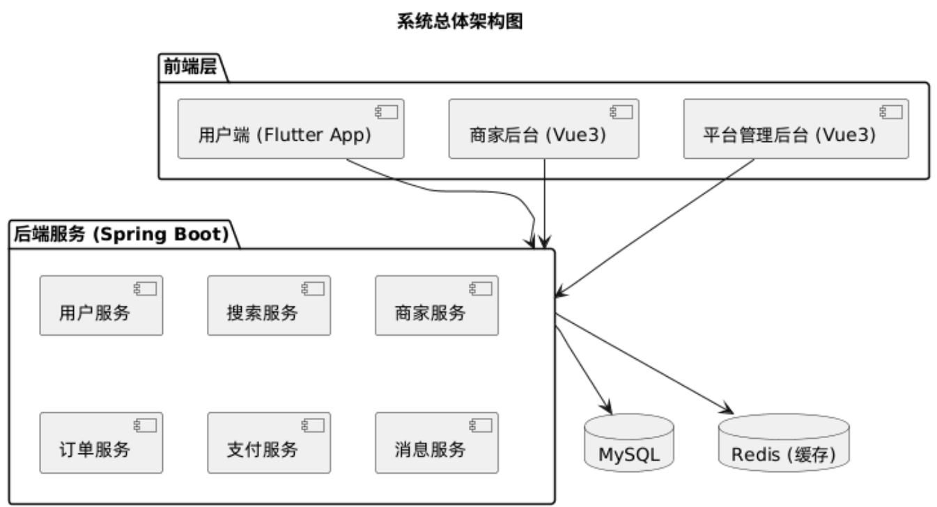
图 2-19 系统总体架构图
