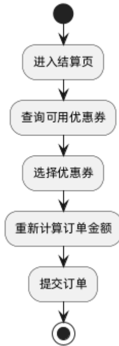
优惠券活动图
