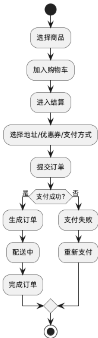
下单活动图（核心流程）
