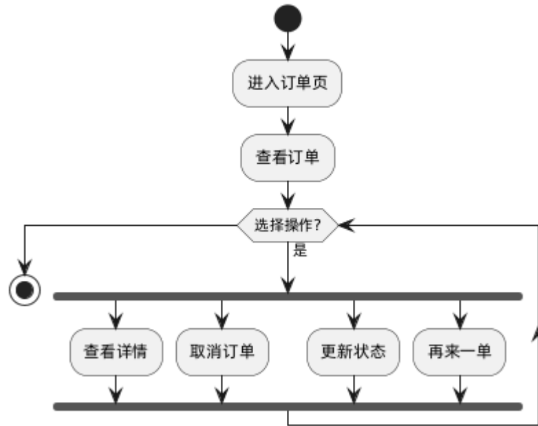
订单管理活动图
