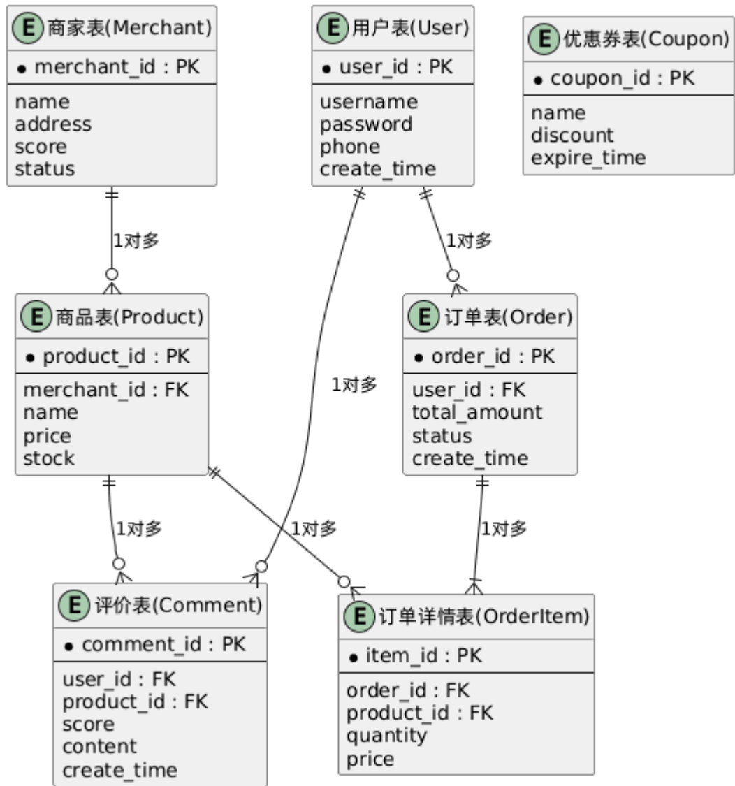
数据库E-R图（简化版）
