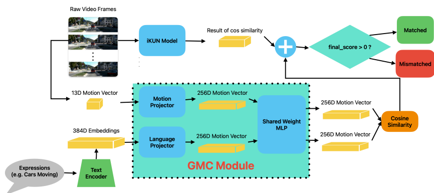
(圖一) GMC-Link 系統架構圖
