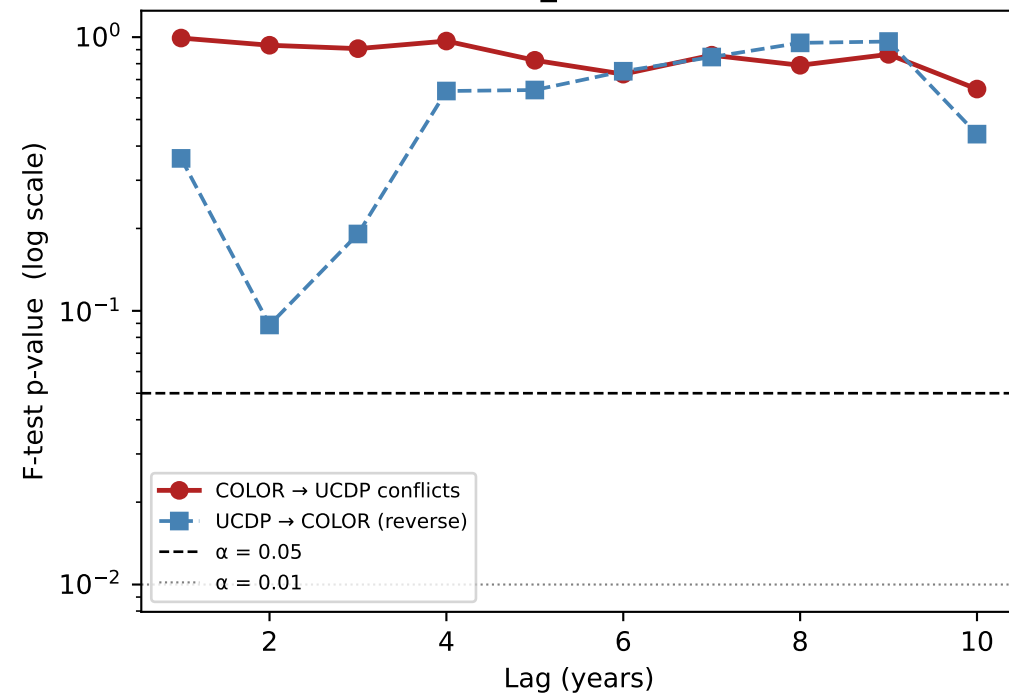
(d) Granger causality [ \Delta UCDP, \Delta COLOR] MAX_LAG=10
