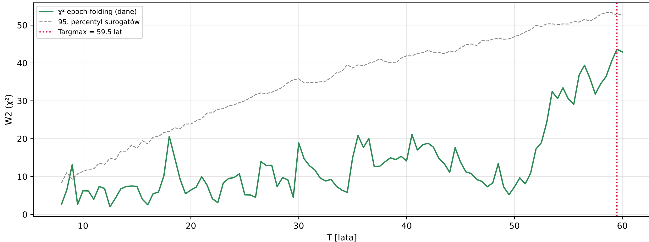
Panel 2. P2 — skan \chi^2 ; Wmax p=0.6152
