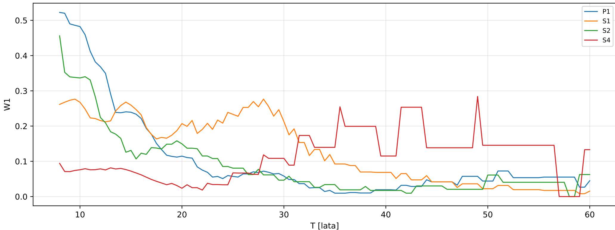
Panel 4. Porównanie serii i okien (W1)
