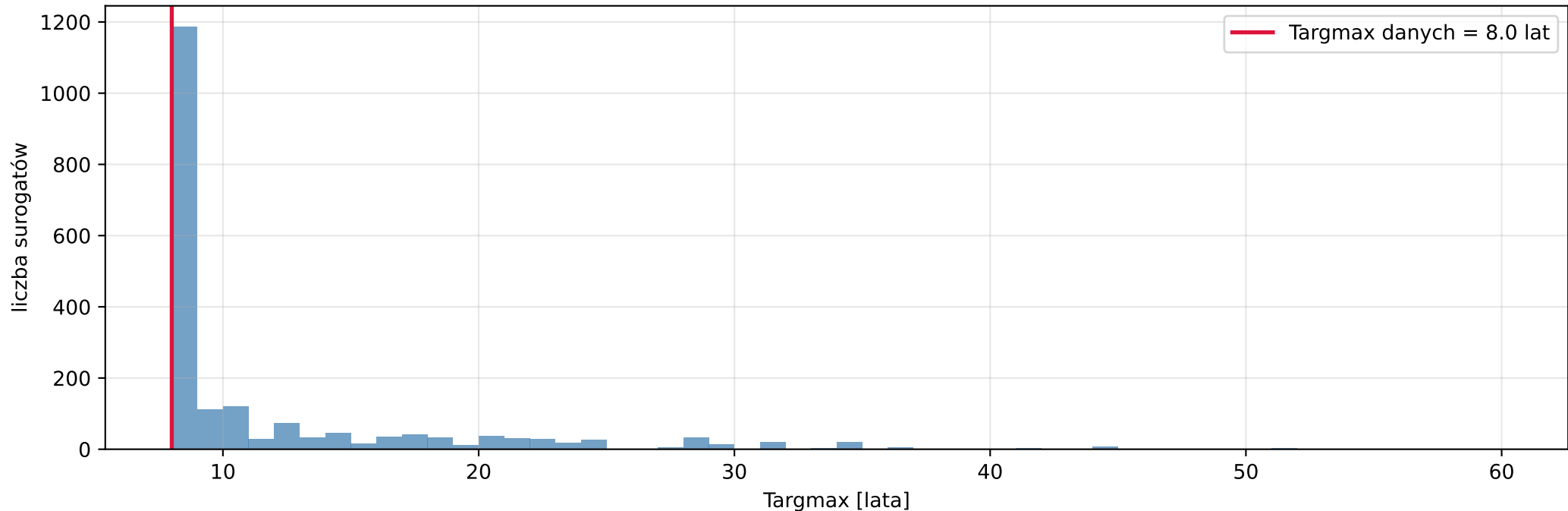
Panel 3. Rozkład Targmax surogatów (kontrola jednorodności, §5/§7)
