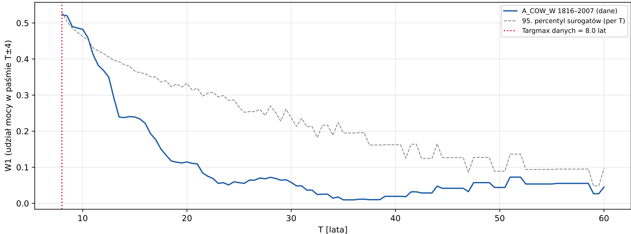
Panel 1. P1 — skan mocy w paśmie; Wmax p=0.0725 (rozkład maksimów)
