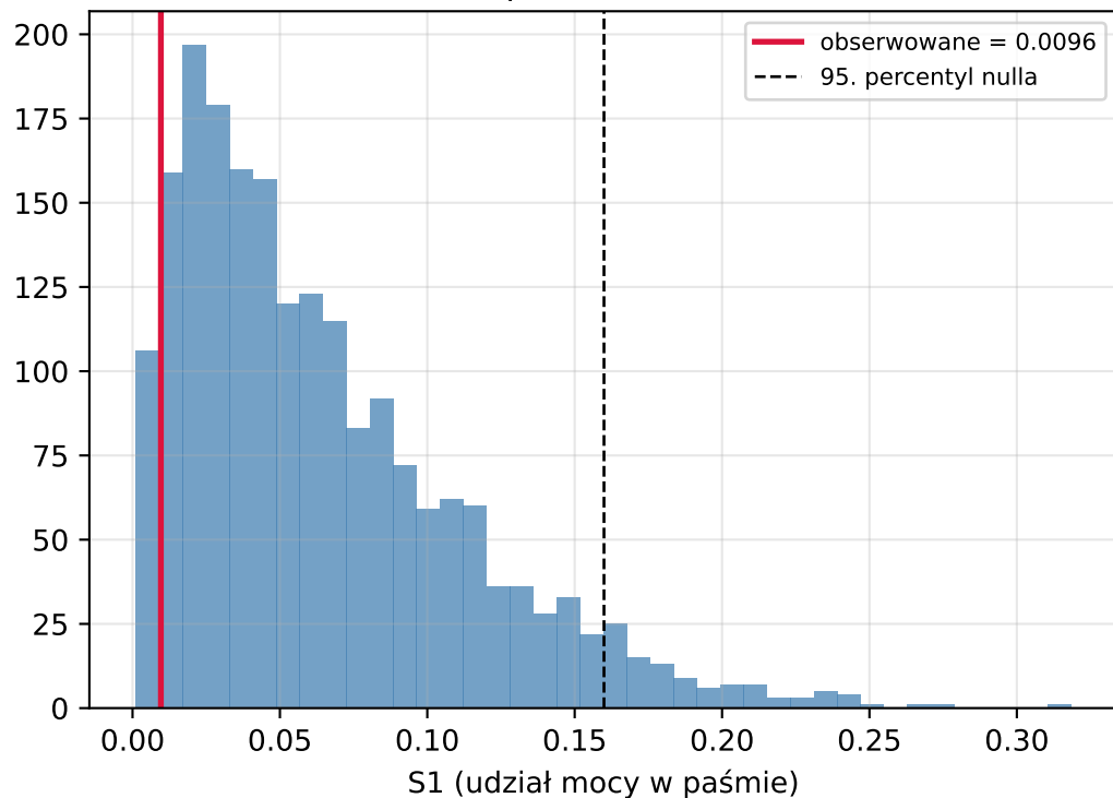
Panel 3b. P2 — null: blok~geom(śr. 10) p = 0.9405
