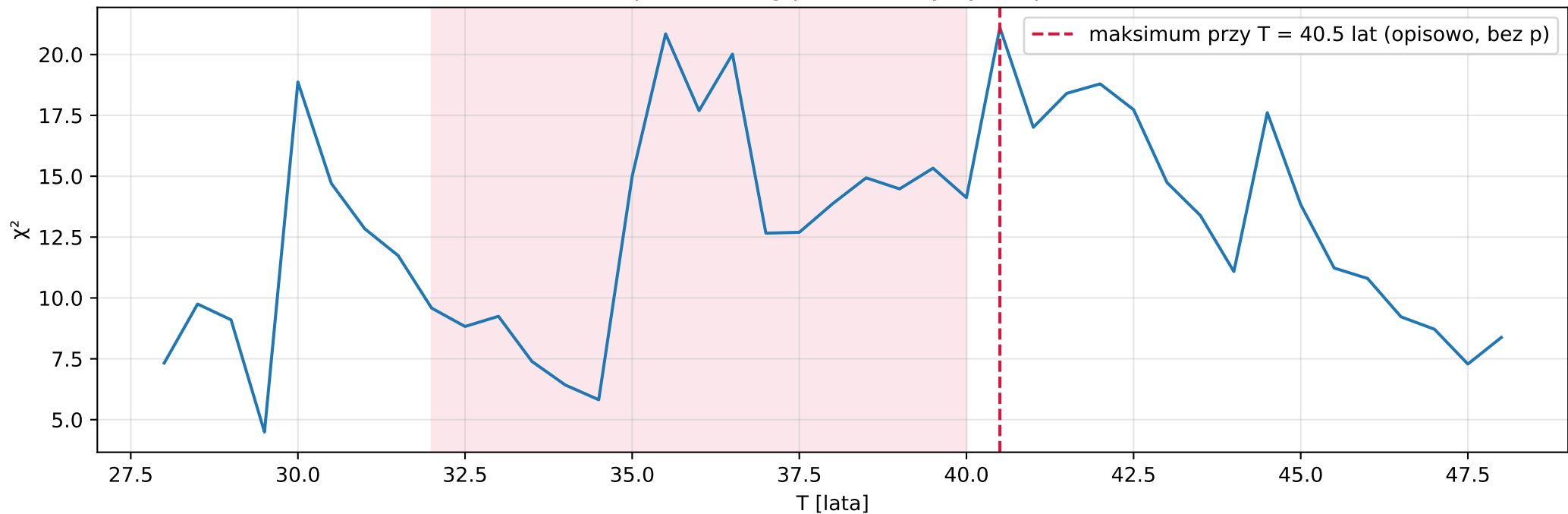
Panel 4. Skan epoch-folding po T — statystyka opisowa (§5, S3)
