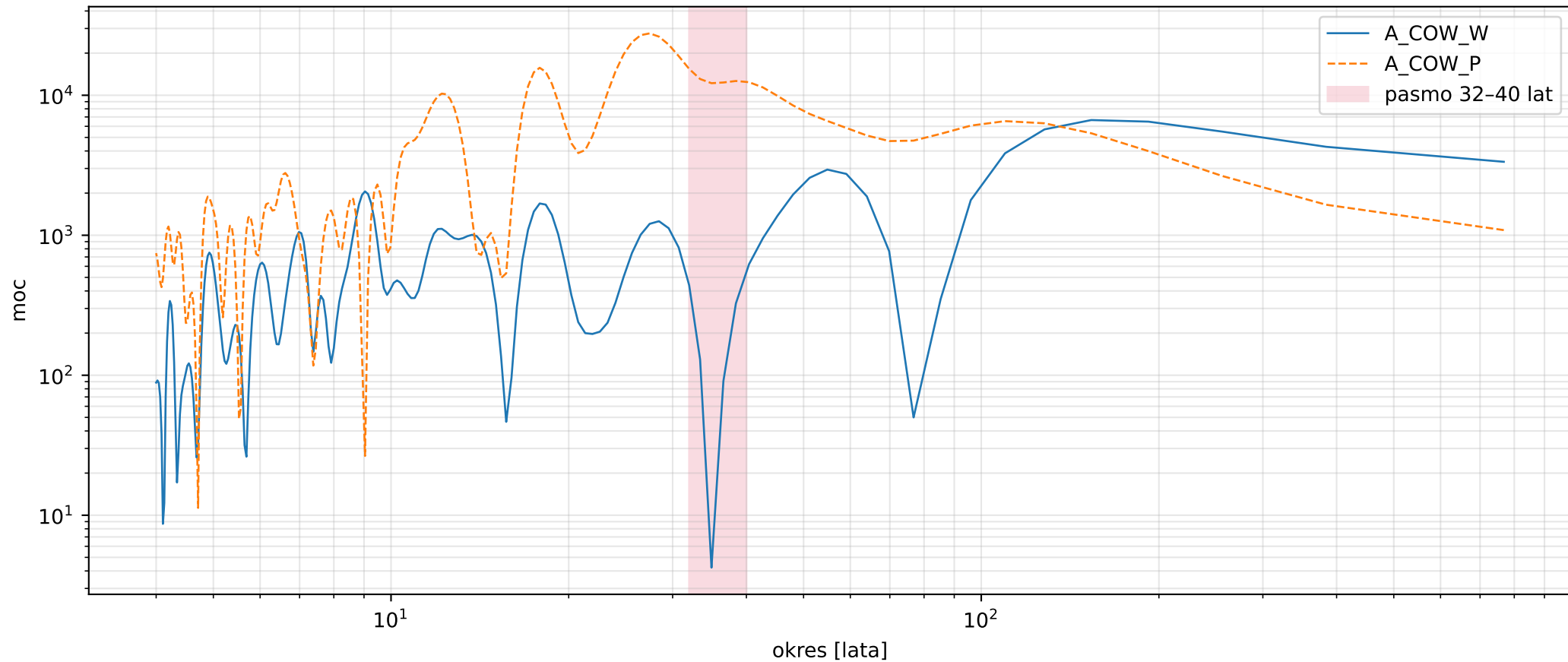
Panel 2. Periodogram (detrend, okno Hanna, uzupełnienie zerami \times 4 )
