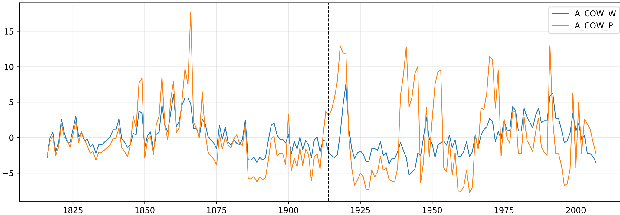
Panel 1b. Te same serie po detrendingu liniowym (1816–2007)
