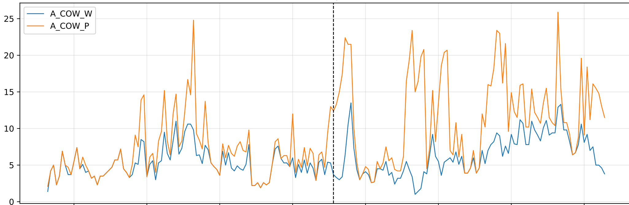
Panel 1a. Serie surowe (pionowa linia: 1914)
