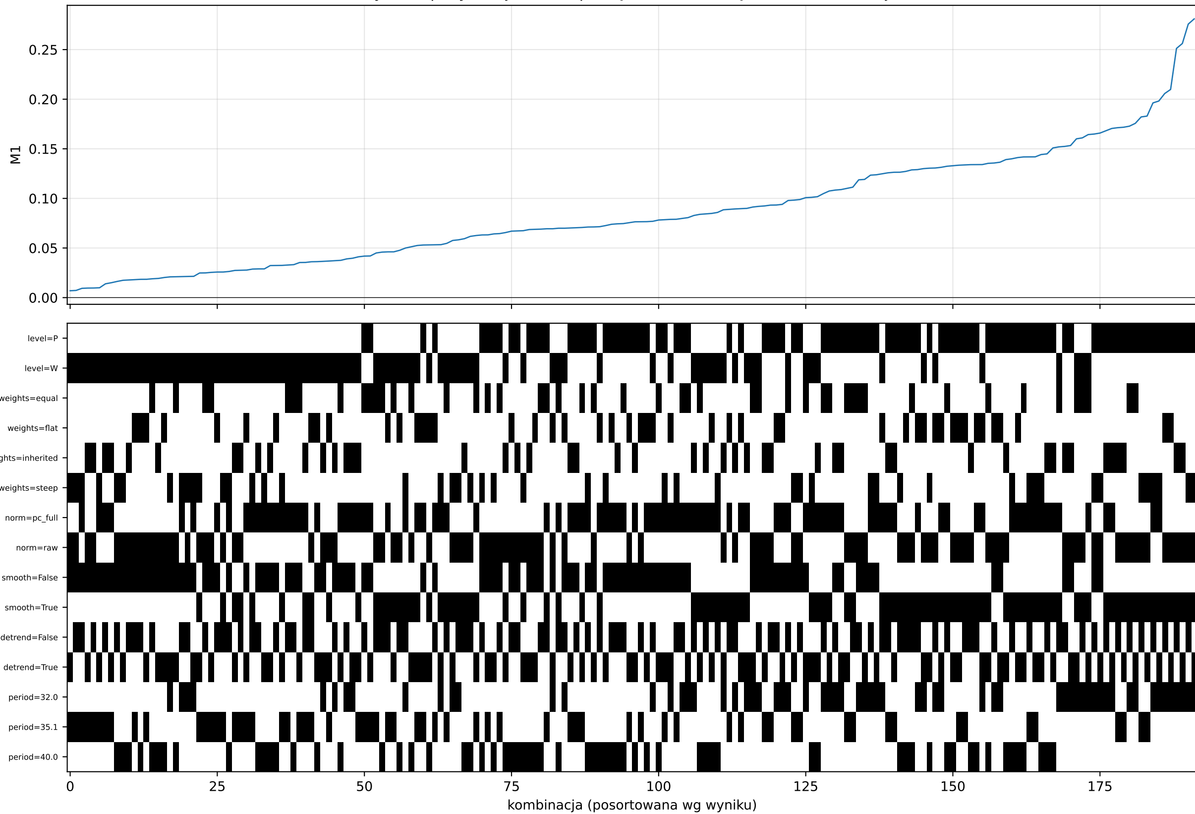
Wykres specyfikacji — M1 uporządkowane rosnąco (192 kombinacje)
