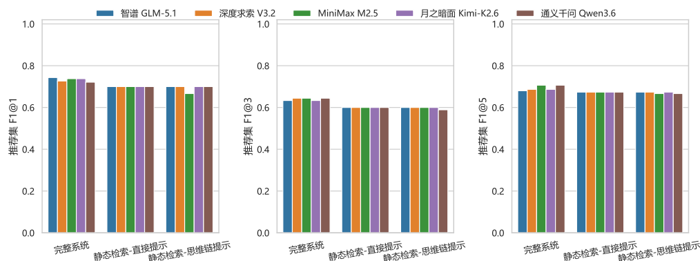
图 4.3: 参考基线横评结果图
